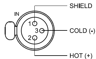
Abbildung 4.5: Belegung AES/EBU-IN
