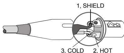
Abbildung 2.12: Symmetrische Beschaltung des Ausgangs (Daisy-Chain)
