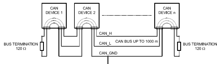
Abbildung 4.10: CAN-Bus mit Linien-Topologie
