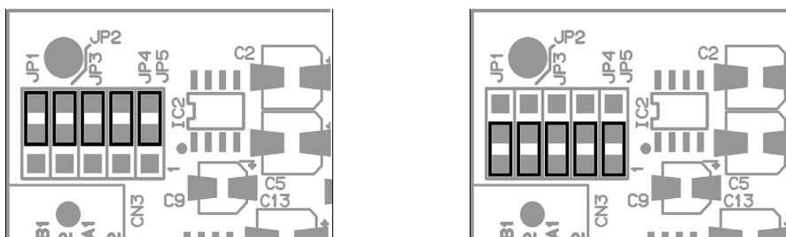
Illustration 4.2: Mode pré-atténuateur (gauche) au mode post-atténuateur (droite)
