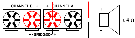
Abbildung 2.17: Lautsprecheranschluss in Betriebsart BRIDGED an Anschlussklemmen
