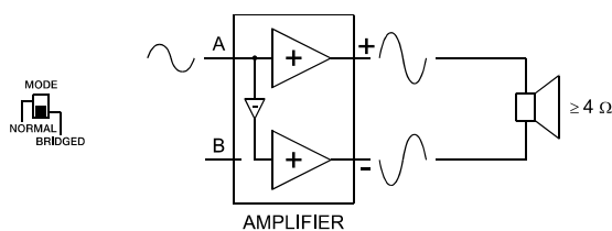
Abbildung 2.9: Betriebsart BRIDGED
