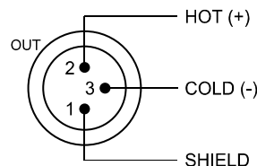
Illustration 4.6: Câblage de la prise AES/EBU-OUT
