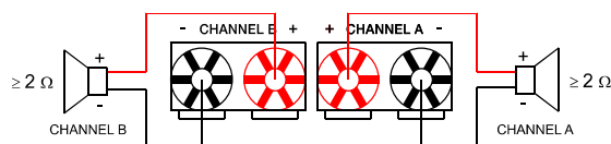
Abbildung 2.14: Lautsprecheranschluss in Betriebsart NORMAL an Anschlussklemmen
