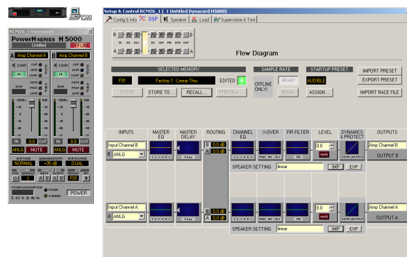
Abbildung 4.3: Bedienpanel und DSP-Flussdiagramm in IRIS-Net
