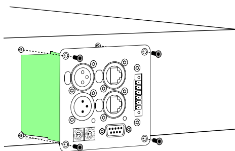
Illustration 4.1: Installation d'un module RCM-26
