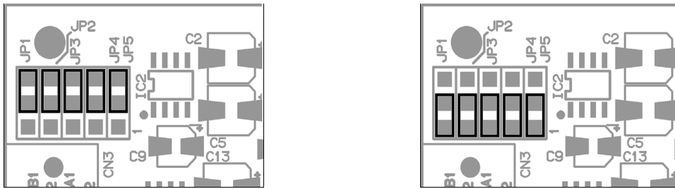
Abbildung 4.2: Jumperstellung in Pre-Fader-Betriebsart (links) und Post-Fader-Betriebsart (rechts)
