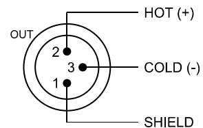
Abbildung 4.6: Belegung AES/EBU-OUT
