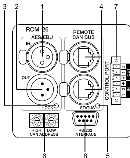
Illustration 4.4: Commandes et connexions RCM-26
