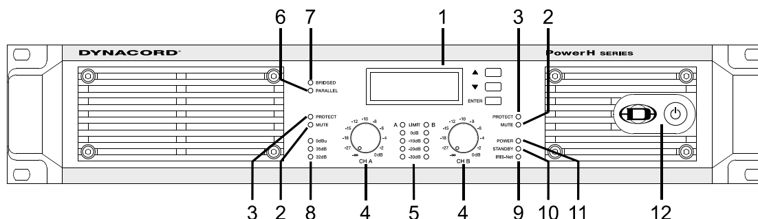
Illustration 2.1 : Face avant du H2500/H5000
