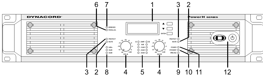
Abbildung 2.1: H2500/H5000 Frontseite
