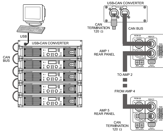
Abbildung 4.11: 5 Remote-Amplifier (mit RCM-26) und ein USB-CAN-Converter am Bus-Anfang. Abschluss-Stecker am USB-CAN-Converter und am RCM-26 des Remote-Amplifier 5
