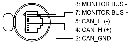
Abbildung 4.7: Belegung der CAN-Buchse
