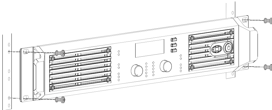
Abbildung 2.4: Vordere Befestigung der Endstufe bei Rackeinbau
