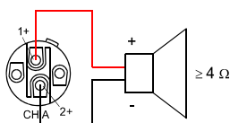
Abbildung 2.16: Lautsprecheranschluss in Betriebsart BRIDGED an Speakon A
