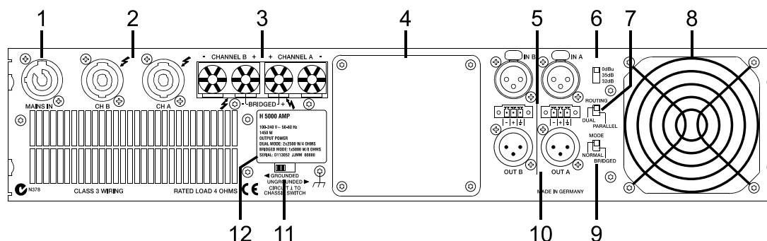
Illustration 2.2 : Arrière du H2500/H5000
