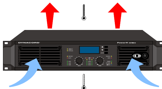
Abbildung 2.6: H2500/H5000 Kühlung
