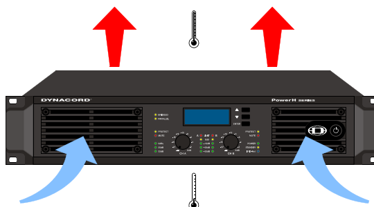
Illustration 2.6 : Refroidissement du H2500/H5000
