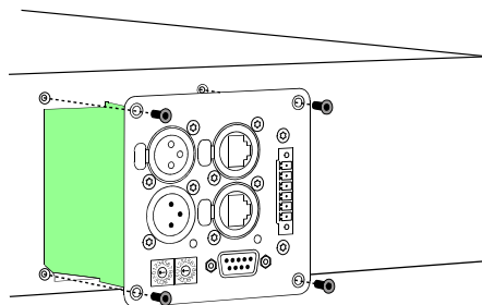
Abbildung 4.1: Einbau des RCM-26 in eine Endstufe
