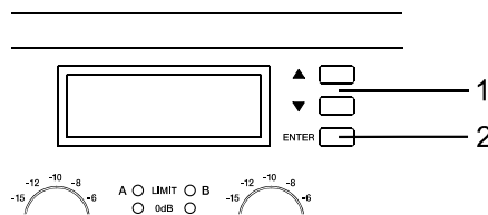
Abbildung 3.2: LC-Display mit Bedienelementen
