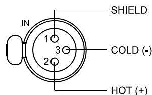
Illustration 4.5: Câblage de la prise AES/EBU-IN
