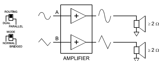
Abbildung 2.7: Einspeisung an beiden Eingängen bei Betriebsart DUAL
