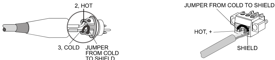
Illustration 2.11 : Connexion non-symétrisé de l'entrée
