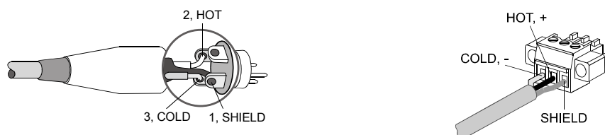
Illustration 2.10 : Connexion symétrisée de l'entrée
