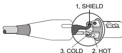
Illustration 2.12 : Connexion symétrisé de la sortie (Daisy-Chain)
