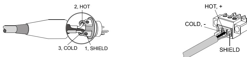
Abbildung 2.10: Symmetrische Beschaltung des Eingangs
