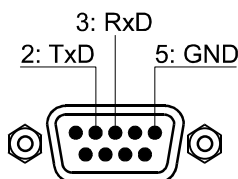
Illustration 4.9: Câblage de l'Interface RS-232
