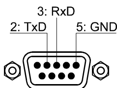
Abbildung 4.9: Belegung der RS-232-Schnittstelle
