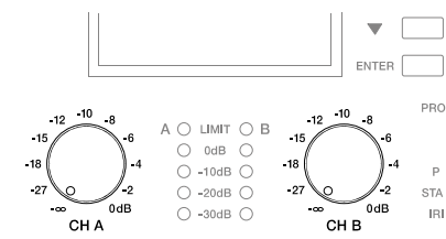
Abbildung 3.1: Levelsteller CH A und CH B
