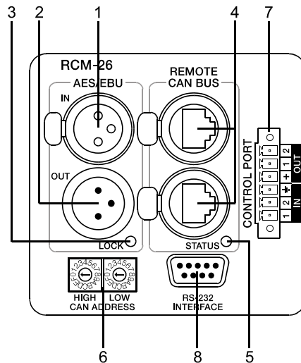
Abbildung 4.4: Bedienelemente und Anschlüsse des RCM-26
