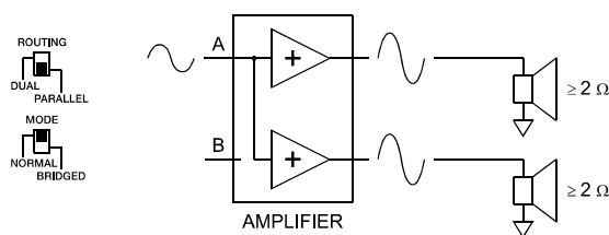
Abbildung 2.8: Einspeisung an Eingang A bei Betriebsart PARALLEL
