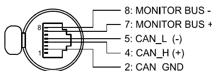
Illustration 4.7: Câblage de la prise CAN
