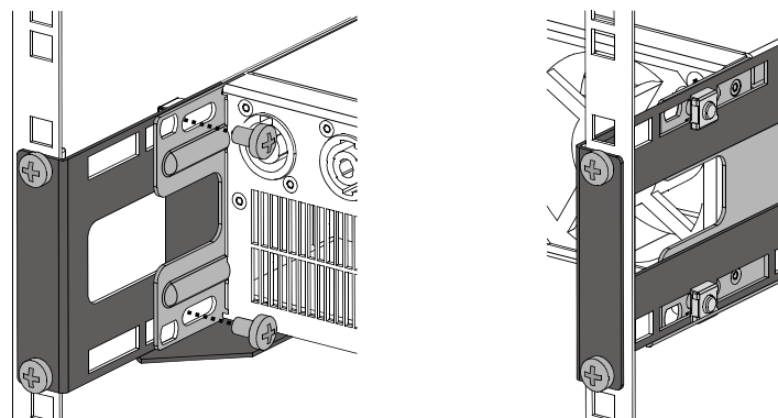
Abbildung 2.5: Hintere Befestigung der Endstufe
